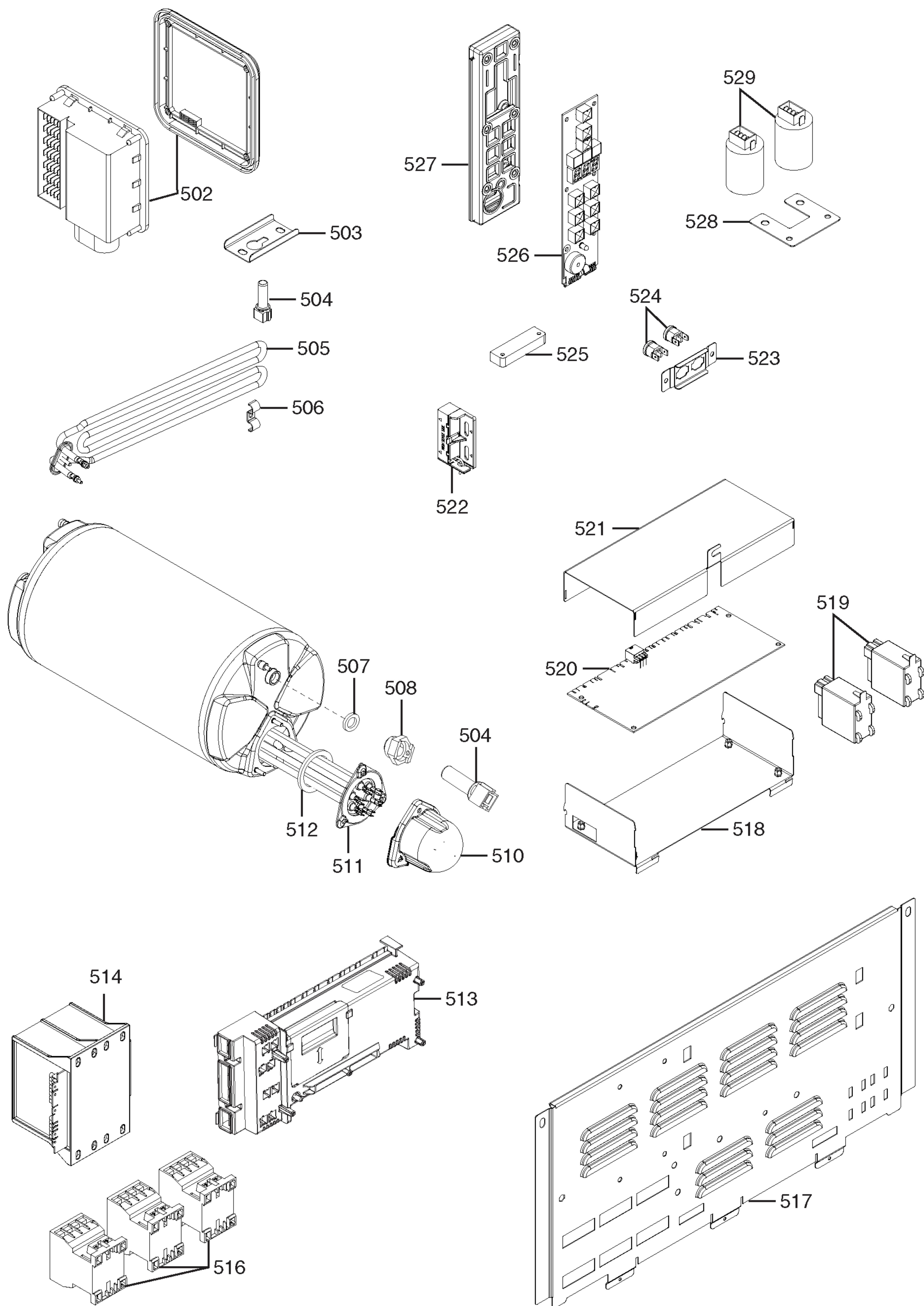
ill. 595668W00_p4 Componenti elettrici / Electrical components
