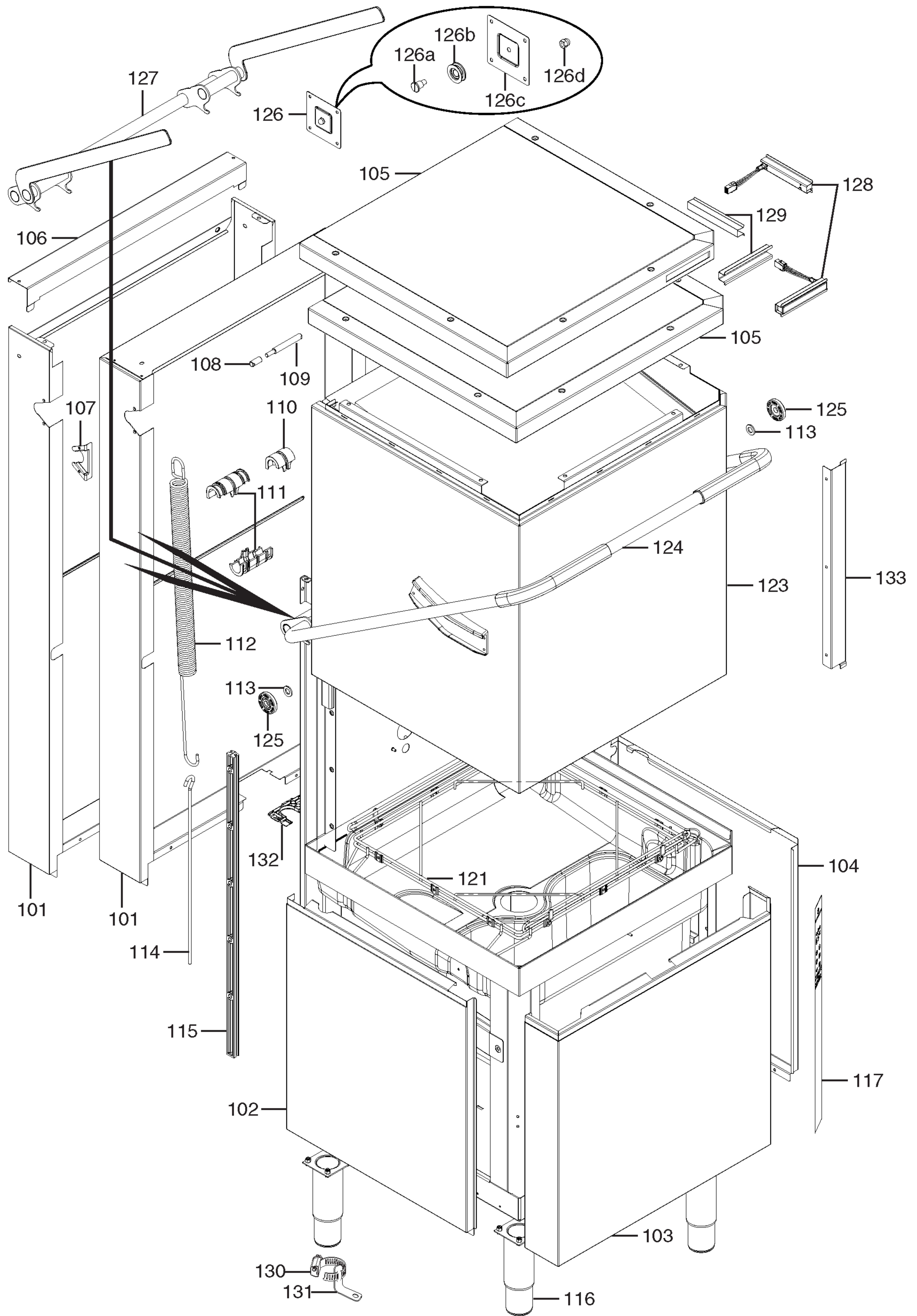
ill. 595668W00_p1 Vista generale / Main view
